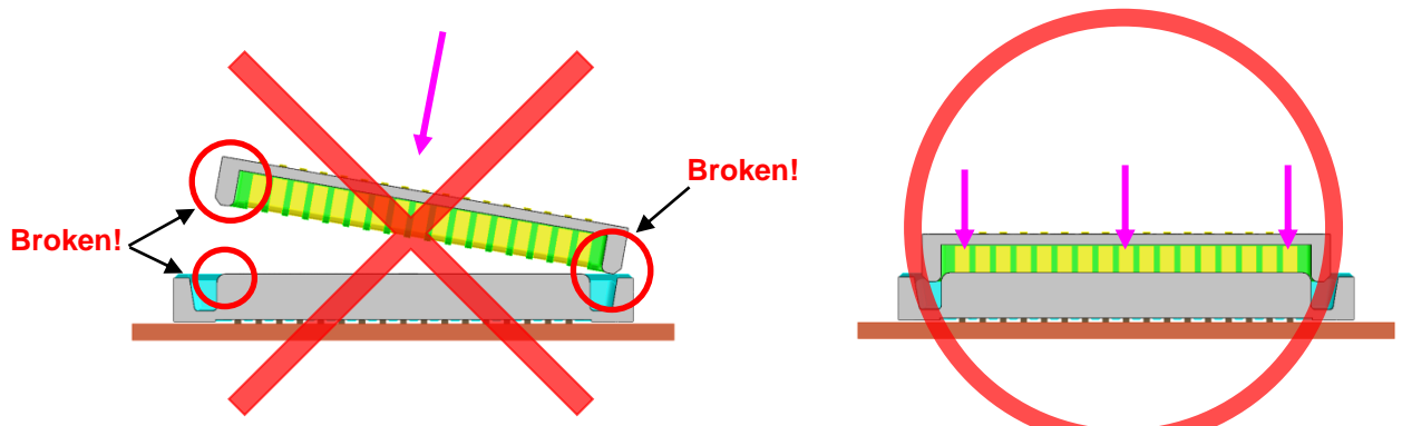
コネクタ斜め嵌合 Mating with angle (Wrong Handling)
