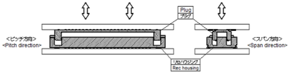
○ 図-1 水平状態での挿抜 Figure-1 Horizontal Mating/Unmating (Best)
