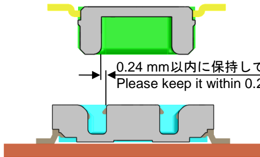
短手方向 "b" Direction
